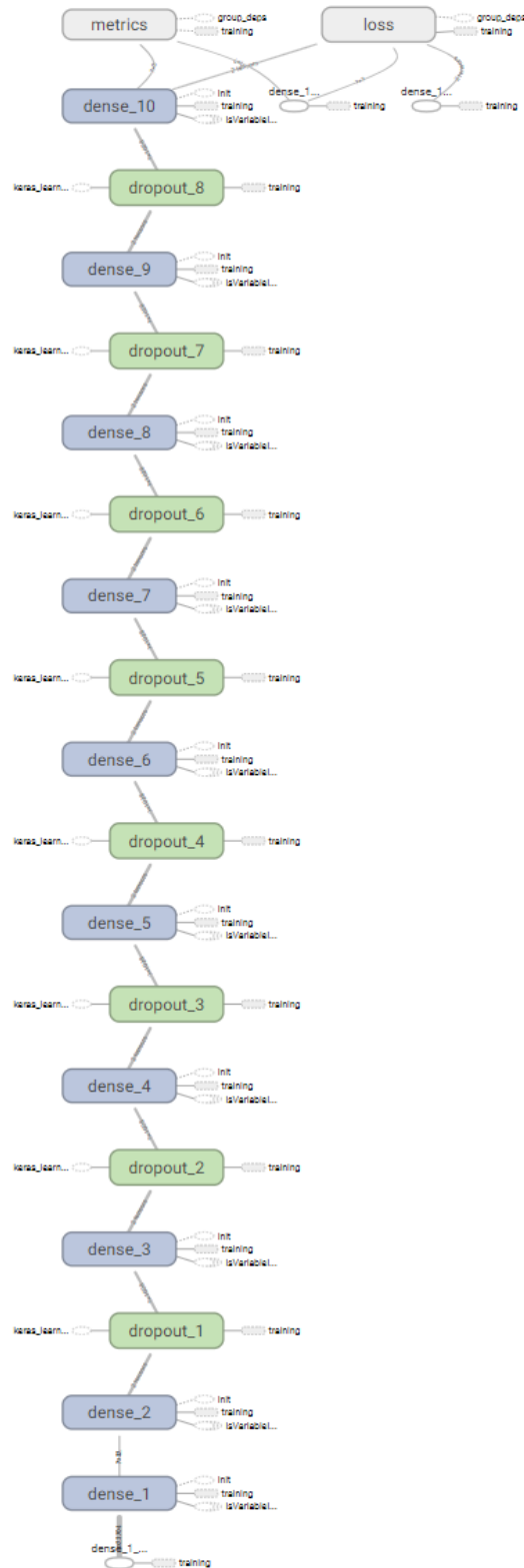
Abbildung D.1: Modellvisualisierung vom HDLTex mittels Tensorboard. Dense 1 repräsentiert den Input-Layer und danach werden die Daten durch 9 KNNs und 8 Dropouts propagiert. Dense 10 stellt den Output-Layer dar. Die genaue Konfiguration ist in Listing D.1 zu sehen.
