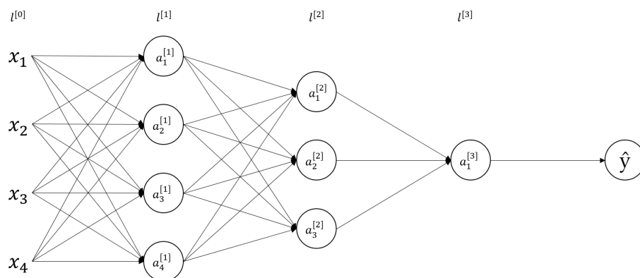
Abbildung 4.8: Diese Abbildung zeigt ein Neuronales Netz mit zwei Hidden Layer. Unser erster Hidden Layer \mathbf{l}^{[1]} besteht aus vier Neuronen n_1 = 4 und der zweite Hidden Layer \mathbf{l}^{[2]} enthält drei Neuronen n_2 = 3 .
