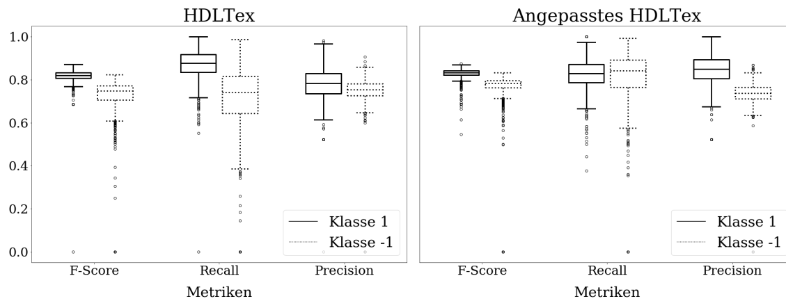
Abbildung 4.13: KNN: Güte. Beide Plots zeigen die Metriken F-Score, Recall und Precision (links das originale HDLTex- und rechts das angepasste HDLTex-Modell).
