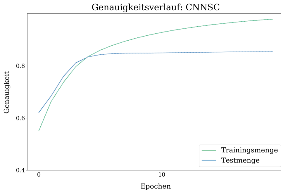
Abbildung D.8: CNNSC: Genauigkeitsverlauf. Die y-Achse repräsentiert die Genauigkeit gegen die Anzahl der Epochen des Trainings (x-Achse). In grün ist die Trainings- und blau die Testmenge zu sehen. Der Plot zeigt eine Vergrößerung der Ansicht des Ergebnisabschnittes 4.16.
