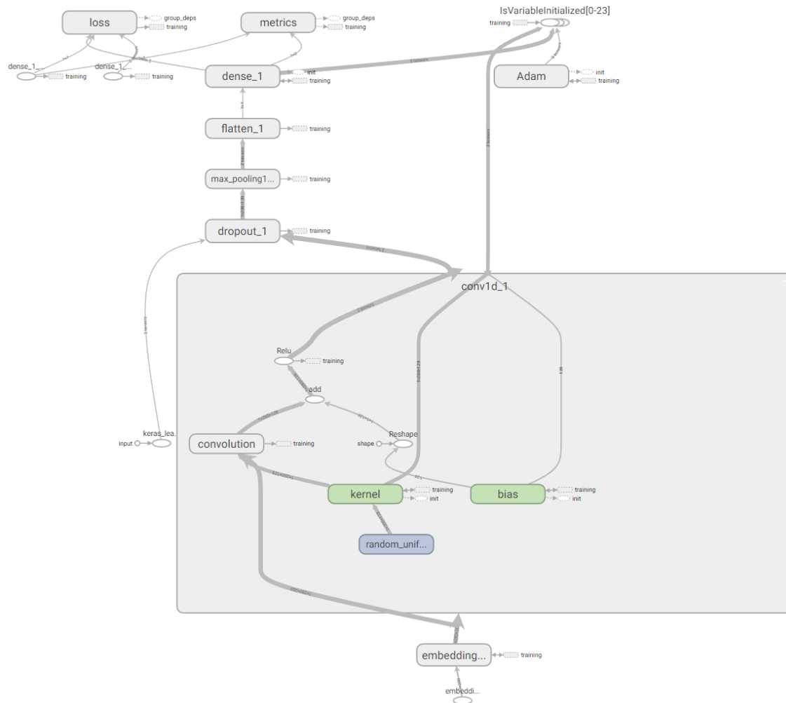
Abbildung D.4: Modellvisualisierung vom angepassten CNNSC mittels Tensorboard. Der Input-Layer ist mittels des Embedding-Layers realisiert. Die graue Box stellt eine detaillierte Ansicht des ersten CNN-Layers dar. Mit Dense 1 ist der Output-Layer gemeint. Die genaue Konfiguration ist im Listing D.4 zu finden.
