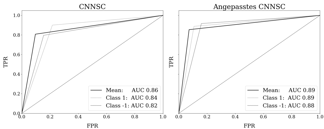
Abbildung 4.18: CNN: ROC-Chart. Der linke Plot zeigt die Ergebnisse als ROC-Chart des originalen HDLTex- und rechts das angepasste Modell.
