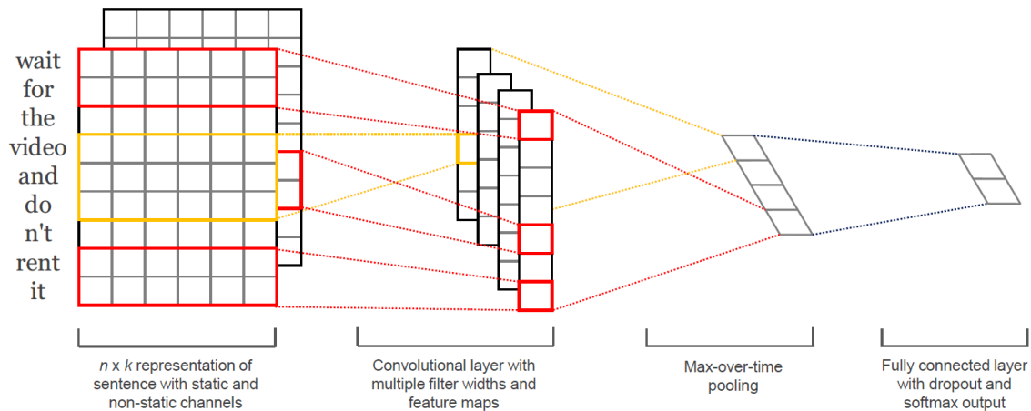
Abbildung 4.15: CNN: Referenzmodell [Kim14, S. 1747]. Beginnend links nach rechts ist der Input eine Gewichtungsmatrix von 300 und der Länge des Vokabulars. Danach folgt der CNN-Layer, Max-Pooling-Layer und das KNN.
