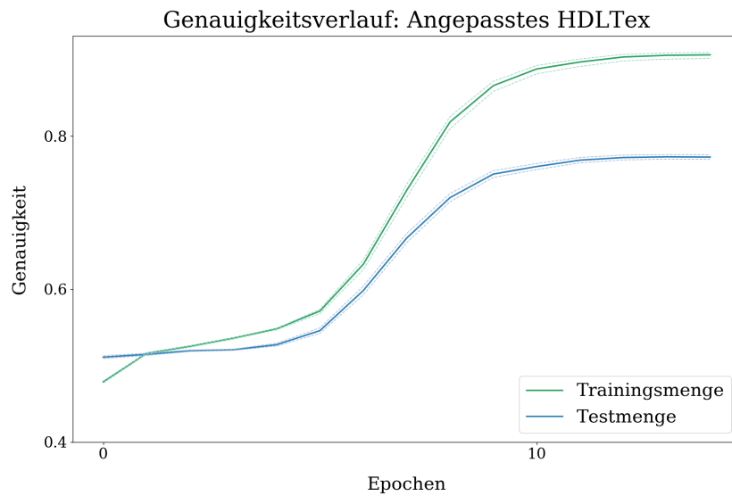
Abbildung D.6: Angepasstes HDLTex: Genauigkeitsverlauf. Die y-Achse repräsentiert die Genauigkeit die Anzahl der Epochen des Trainings (x-Achse). In grün ist die Trainings- und blau die Testmenge zu sehen. Der Plot zeigt eine Vergrößerung der Ansicht des Ergebniskapitels 4.12.
