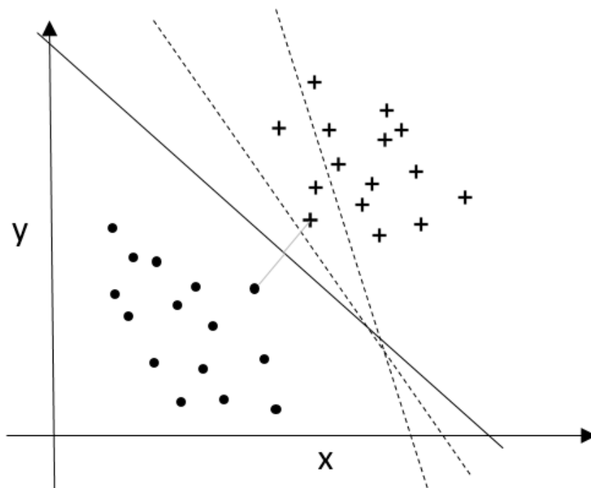
Abbildung C.3: Beispiel für ein Support Vector Machine Klassifikation. Die durchgezogene Hyperebene trennt die zwei Klassen mit einem maximalen Margin, wohingegen die gestrichelten Hyperebenen sie trennen, aber nicht perfekt. Die Objekte, die die Hyperebene bilden, werden Support Vektoren genannt.
