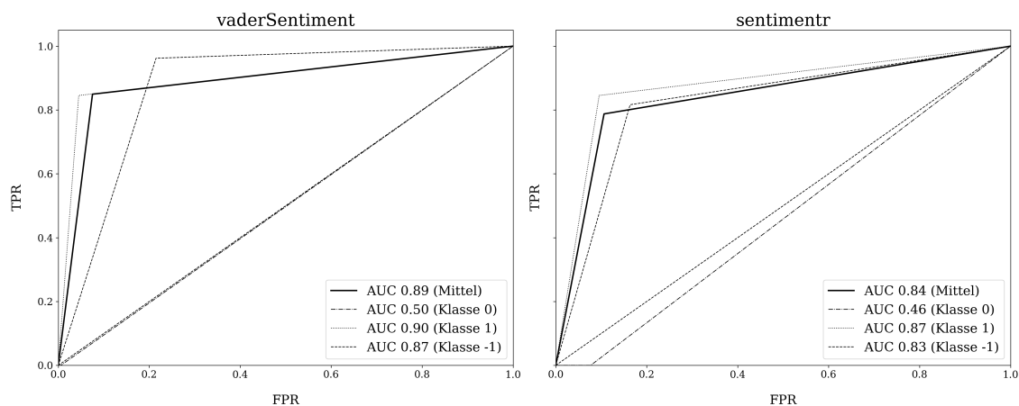
Abbildung C.1: ROC-Charts der lexikalischen Methoden. Der linke ROC-Chart zeigt das Ergebnis vom vaderSentiment und rechts sentimentr.
