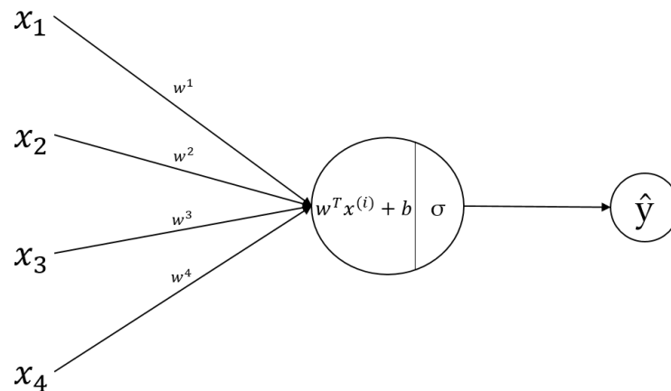
Abbildung 4.4: Ein Neuronales Netz mit vier Inputs, einem Hidden Layer mit einem Neuron, bzw. Perzeptron, und einem Output.
