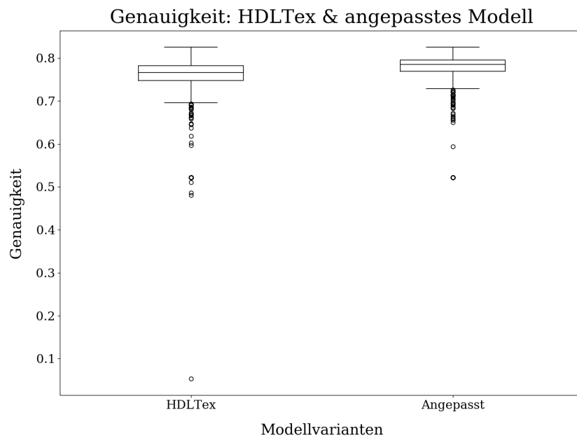
Abbildung D.7: Diese Abbildung stellt die Ergebnisse, hier die Genauigkeit, des HDLTex-Modells dem angepassten Modell gegenüber. Der linke Boxplot zeigt die Verteilung für das HDLTex-Modell und rechts unser angepasstes Modell über 1.000 Modelle an.
