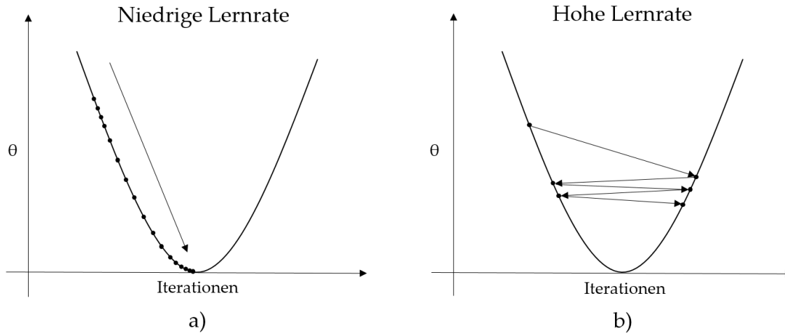
Abbildung 4.6: Auswirkung des Parameters Lernrate auf das Lernverhalten. Die x-Achse spiegelt die Anzahl der Iterationen und die y-Achse die Lernrate wieder. a) Die Lernrate ist gut eingestellt und konvergiert gegen das optimale Modell. b) Die Lernrate ist zu hoch eingestellt und die Gefahr der Divergenz besteht.
