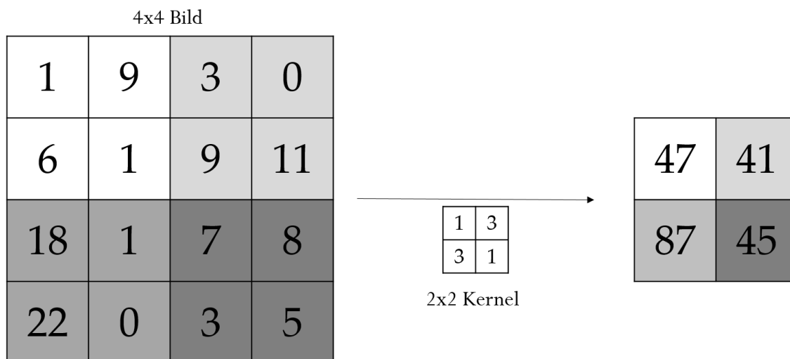
Abbildung 4.9: Einfaches CNN Beispiel (Pooling). Auf der linken Seite erhält das CNN ein 4 \times 4 Bild. Die Graustufen spiegeln die Fenster wieder, indem der 2 \times 2 Kernel Berechnungen durchführt. Der Kernel iteriert über das Bild in zweier Schritten, \text{stride} = 2 , von links nach rechts und von oben nach unten. Als Ergebnis erhalten wir wiederum eine 2 \times 2 Matrix. Die Berechnung für die weiße Fläche könnte wie folgt aussehen: 1 * 1 + 9 * 3 + 6 * 3 + 1 * 1 .
