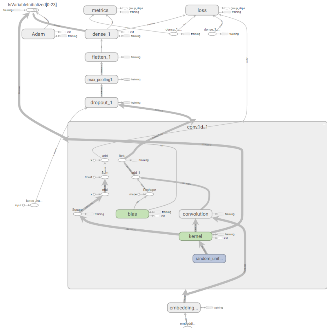
Abbildung D.3: Modellvisualisierung vom CNNSC mittels Tensorboard. Der Input-Layer ist mittels dem Embedding-Layer realisiert. Die graue Box stellt eine detaillierte Ansicht des ersten CNN-Layers dar. Mit Dense 1 ist der Output-Layer gemeint. Die genaue Konfiguration ist im Listing D.3 zu finden.
