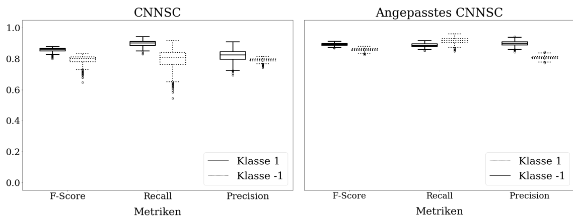
Abbildung 4.17: CNN: Güte. Beide Plots zeigen die Metriken F-Score, Recall und Precision (links das originale CNNSC- und rechts das angepasste CNNSC-Modell).
