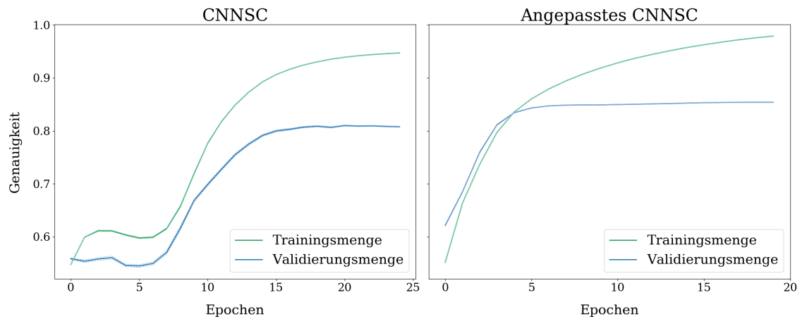
Abbildung 4.16: CNN: Verlauf der Genauigkeit. Der linke Plot zeigt das originale CNNSC Modell aus “Convolutional Neural Networks for Sentence Classification” [Kim14, S. 1748]. Rechts ist unser angepasstes Modell zu sehen.
