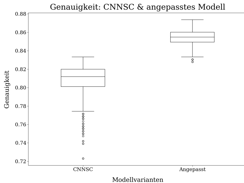
Abbildung D.10: Diese Abbildung stellt die Ergebnisse, hier die Genauigkeit, des CNNSC-Modells gegenüber des angepassten Modells. Der linke Boxplot zeigt die Verteilung für das CNNSC-Modell und rechts unser angepasstes Modell über 1.000 Modelle an.
