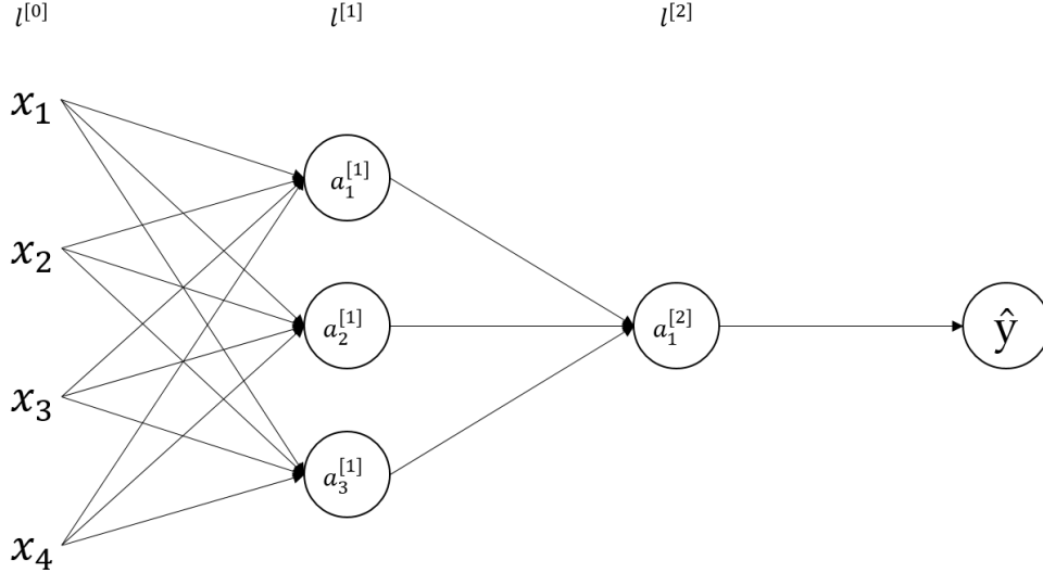
Abbildung 4.7: Das Neuronale Netz besteht aus L = 2 Layer. Der Hidden Layer l^{[1]} besteht aus n_1 = 3 Neuronen. a_{n_1} bezeichnet das Ergebnis eines Neurons mit der Aktivierungsfunktion.
