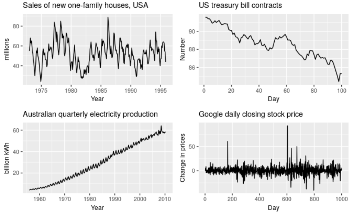
Abbildung 5.1: Komponenten der Zeitreihen [Hyn14, Abbildung 2.3]. Links oben repräsentiert die Verkäufe von Einfamilienhäuser in den USA und zeigt starke saisonale und zyklische (6-10 Jahre) Muster auf, jedoch keinen Trend. Rechts oben zeigt die Staatsanleihe von der United States, die lediglich einen Abwärtstrend aufweist. Links unten zeigt die Produktion von Strom in Australien, die einen steigenden Trend mit einem starken saisonalen Effekt aufweist. Rechts unten werden die Aktienpreise von Google angezeigt, die keine Effekte aufzeigen.
