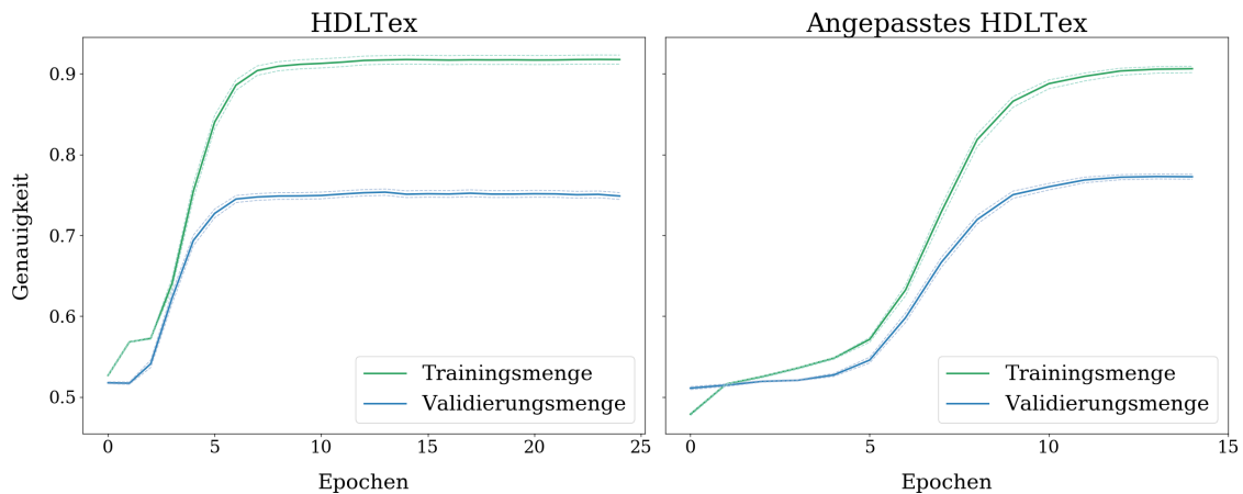
Abbildung 4.12: KNN: Verlauf der Genauigkeit. Der linke Plot repräsentiert den Genauigkeitsverlauf über 25 Epochen des originalen Modells [Kow17, S. 5]. Der rechte Plot zeigt den Verlauf für unser angepasstes Modell.
