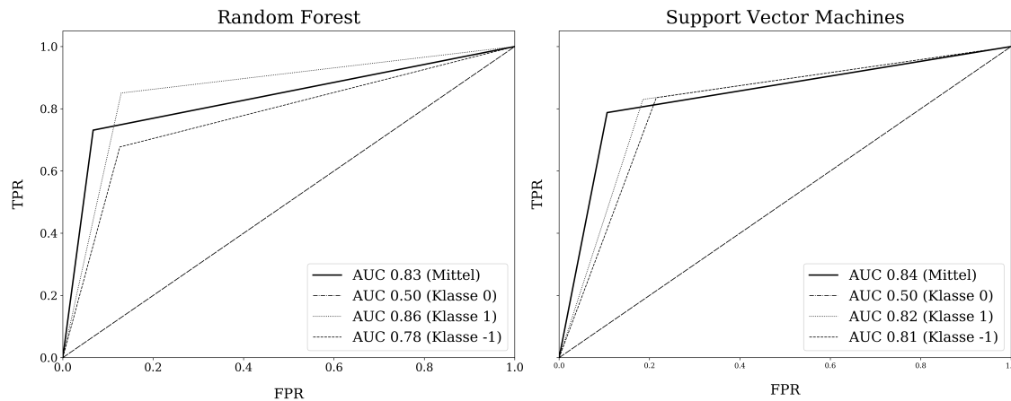
Abbildung C.4: ROC-Charts der maschinellen Lernmethoden. Der linke ROC-Chart zeigt das Ergebnis von Random Forest und rechts von den Support Vector Machines.
