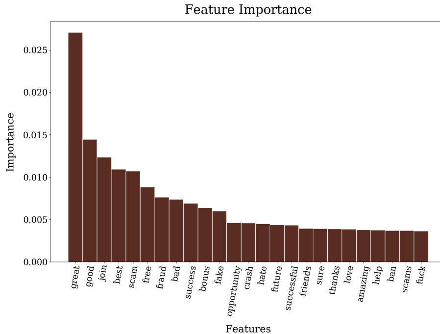
Abbildung 3.2: FI mit Datenvorbereitung (Entfernen von Kleinschreibung, Stoppwörter, Hashtags, HTML-Code, URLs, Nutzer und Eigennamen).
