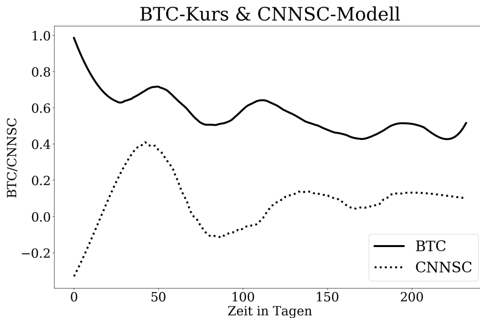
Abbildung 1.1: BTC-Kurs und CNNSC-Modell. Die x-Achse repräsentiert die Tage in einem Zeitraum vom 10.01. - 31.08.2018 und die y-Achse das Bitcoin-Niveau und dem errechneten Sentiment vom CNNSC-Modell.
