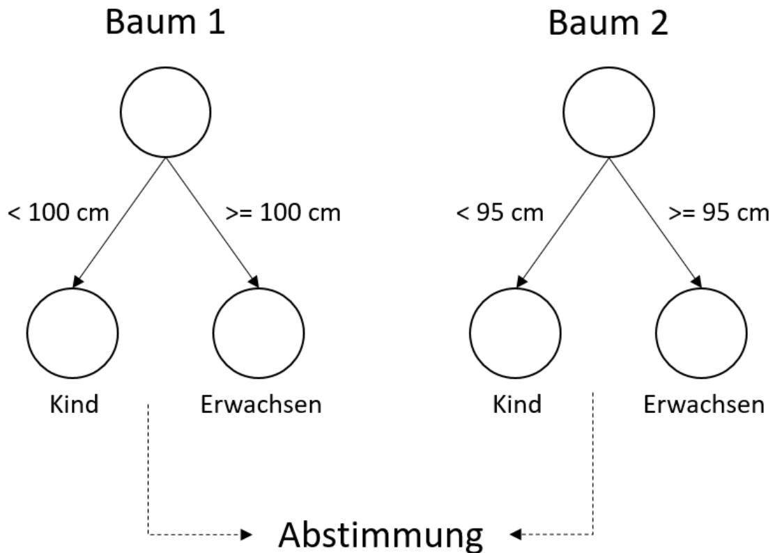
Abbildung C.2: Beispiel für einen Random Forest. In diesem Fall besteht der RF aus zwei Entscheidungsbäumen, die jeweils versuchen einen Menschen anhand der Körpergröße in die Klassen Kind oder Erwachsener einzuteilen. Der Threshold für Baum 1 liegt bei 100 cm und für Baum 2 bei 95 cm. Nachdem die beiden Bäume eine Entscheidung getroffen haben, werden diese einen Mehrheitsvotum unterzogen.
