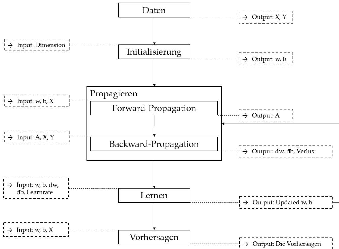
Abbildung 4.5: Schematischer Ablauf eines Lern-Algorithmus
