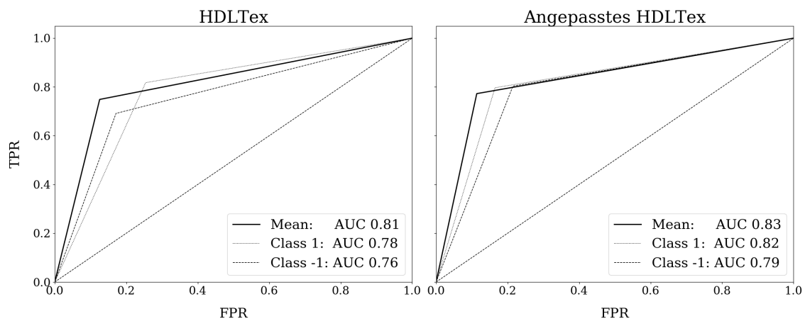
Abbildung 4.14: KNN: ROC-Chart. Der linke Plot zeigt die Ergebnisse als ROC-Chart des originalen HDLTex- und rechts das angepasste Modell.
