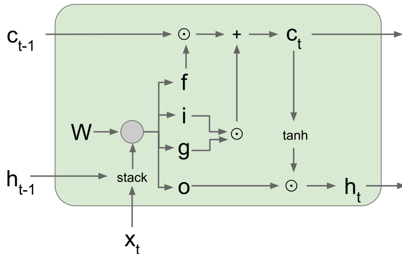
Abbildung 4.11: Die Abbildung zeigt den Aufbau einer LSTM-Zelle [Li18, Folie 10-98]. Von links nach rechts werden die Daten propagiert. c_{t-1} und c_t stellen den vorigen und jetzigen Zellstatus dar. h_{t-1} und h_t repräsentieren den vorigen und jetzigen versteckten Zellstatus. x_t ist unser Datenpunkt, W die Gewichtungsmatrix und mit f (Forget), i (Input), g (Gate) und o (Output) repräsentieren wir die Gates.
