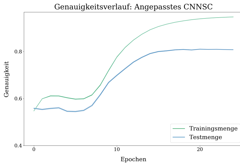
Abbildung D.9: Angepasstes CNNSC: Genauigkeitsverlauf. Die y-Achse repräsentiert die Genauigkeit gegen die Anzahl der Epochen des Trainings (x-Achse). In grün ist die Trainings- und blau die Testmenge zu sehen. Der Plot zeigt eine Vergrößerung der Ansicht des Ergebnisabschnittes 4.16.
