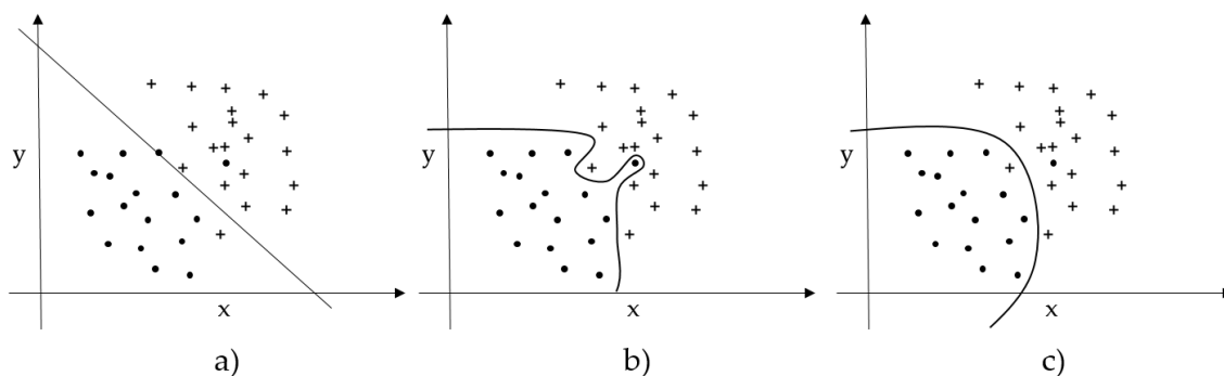
Abbildung 4.3: Die drei Plots zeigen den Bias-Varianz-Tradeoff. a) enthält einen hohen Bias und eine niedrige Varianz. b) zeigt einen niedrigen Bias, jedoch eine hohe Varianz. c) illustriert einen ausgeglichenen Bias und Varianz.
