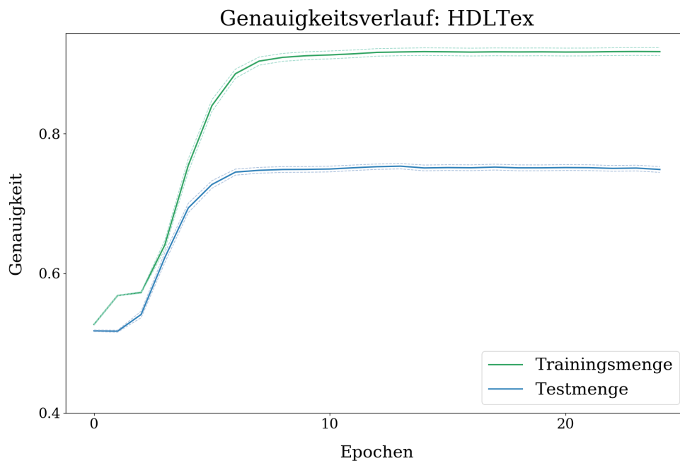
Abbildung D.5: HDLTex: Genauigkeitsverlauf. Die y-Achse repräsentiert die Genauigkeit gegen die Anzahl der Epochen des Trainings (x-Achse). In grün ist die Trainings- und blau die Testmenge zu sehen. Der Plot zeigt eine Vergrößerung der Ansicht des Ergebnisabschnittes 4.12.
